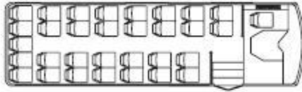
604 • 31-passenger
