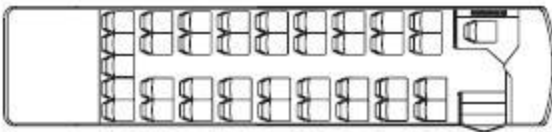
703 • 37-passenger
